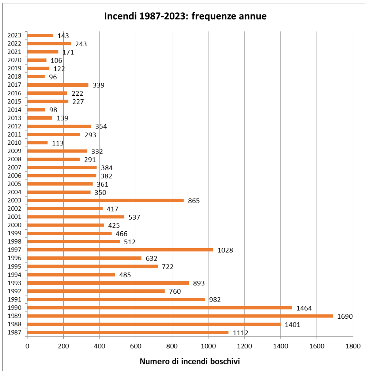
Figura 32. Evoluzione temporale del numero di incendi annuale.
