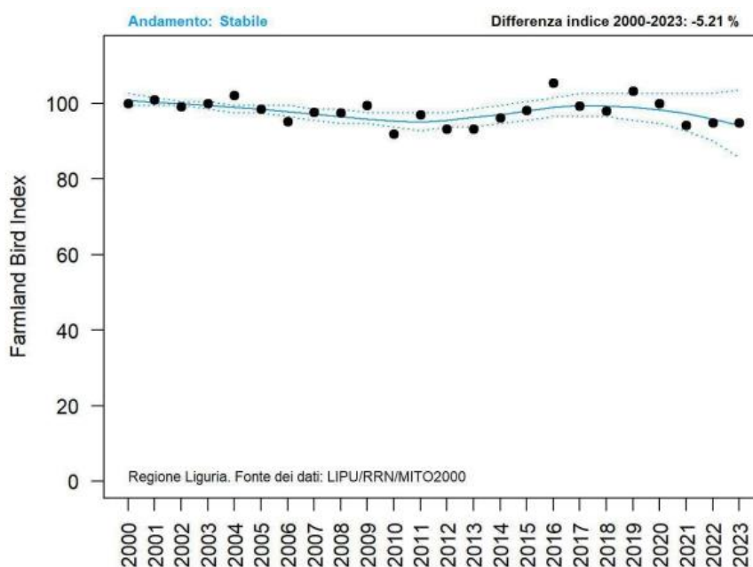
Figura 7. Andamento del Farmland Bird Index regionale nel periodo 2000-2023. I punti indicano i valori annuali del FBI (calcolato come media geometrica degli andamenti delle singole specie), la linea continua e le linee tratteggiate rappresentano rispettivamente la tendenza dell'indice ed il relativo intervallo di confidenza al 95% (stimati con MSI-tool) Fonte: Rete Rurale Nazionale & Lipu – Farmland Bird Index e andamenti di popolazione delle specie 2000-2023 - Liguria.
