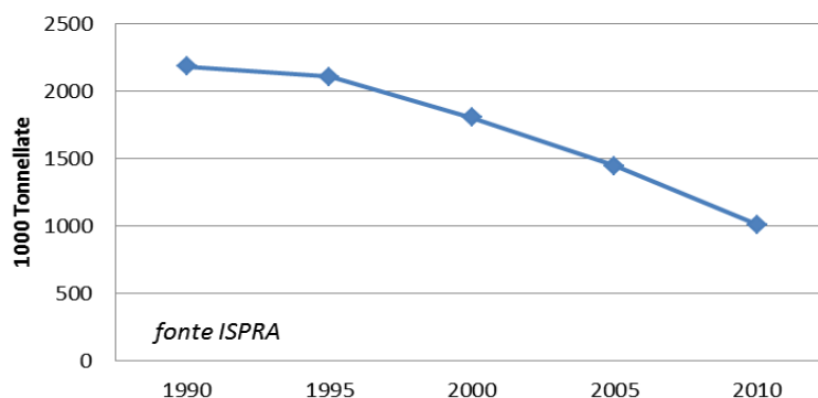
Figura 22. Emissione di gas a effetto serra in agricoltura in migliaia di tonnellate.
