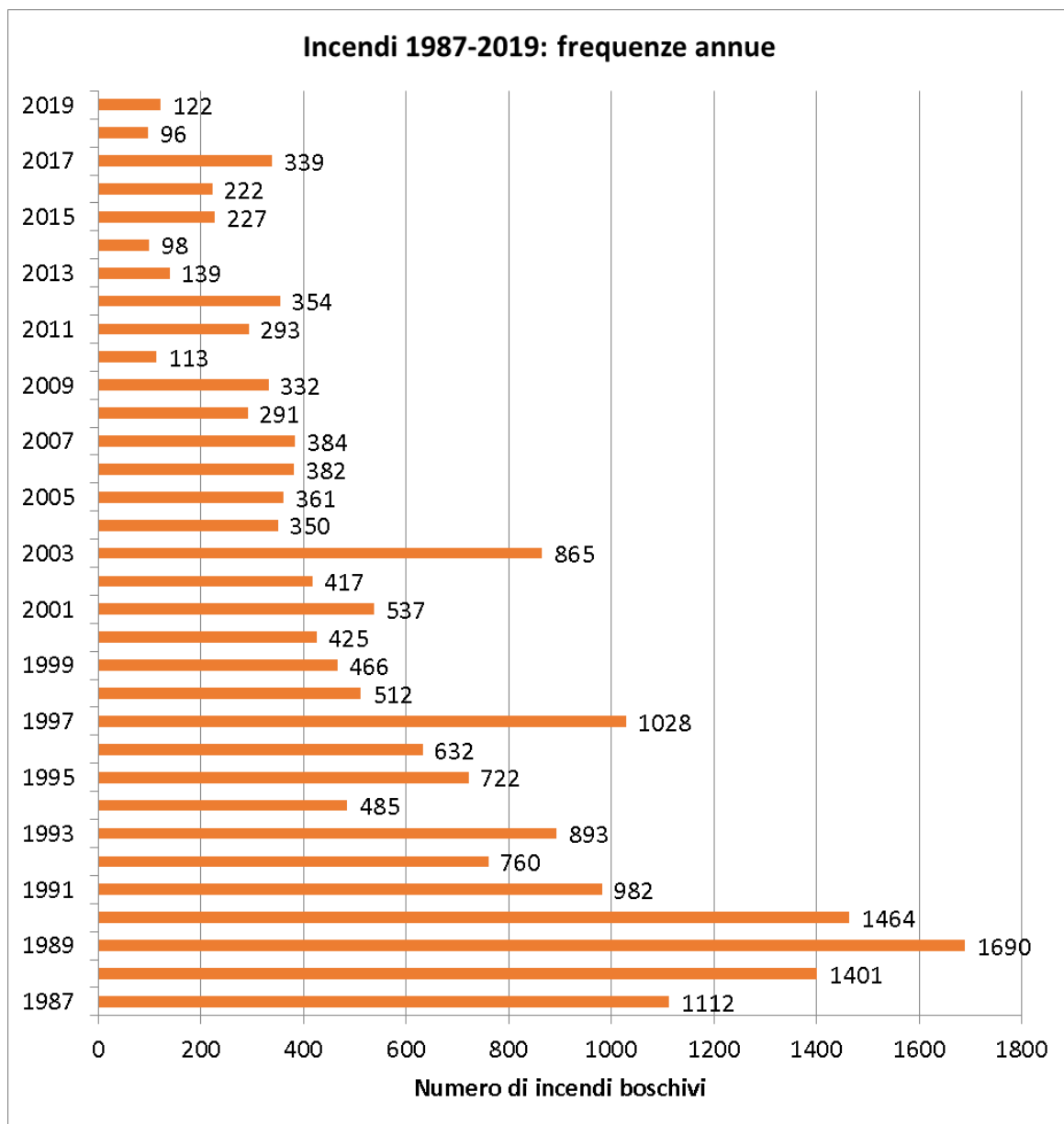
Figura 31. Evoluzione temporale del numero di incendi annuale.
