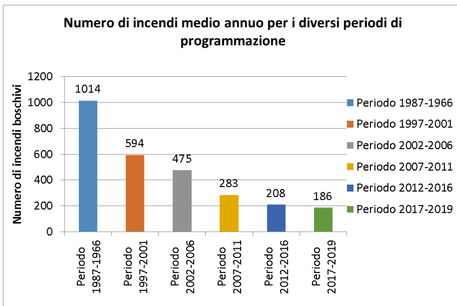
Figura 30. Numero medio di incendi nel periodo considerato.
