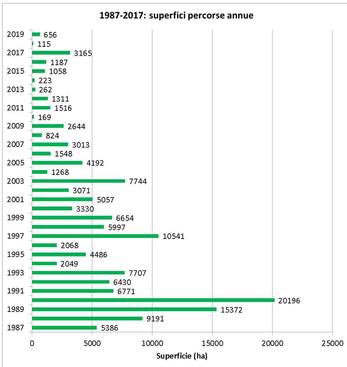
Figura 32. Evoluzione storica della superficie percorsa da incendi, espressa in ettari.
