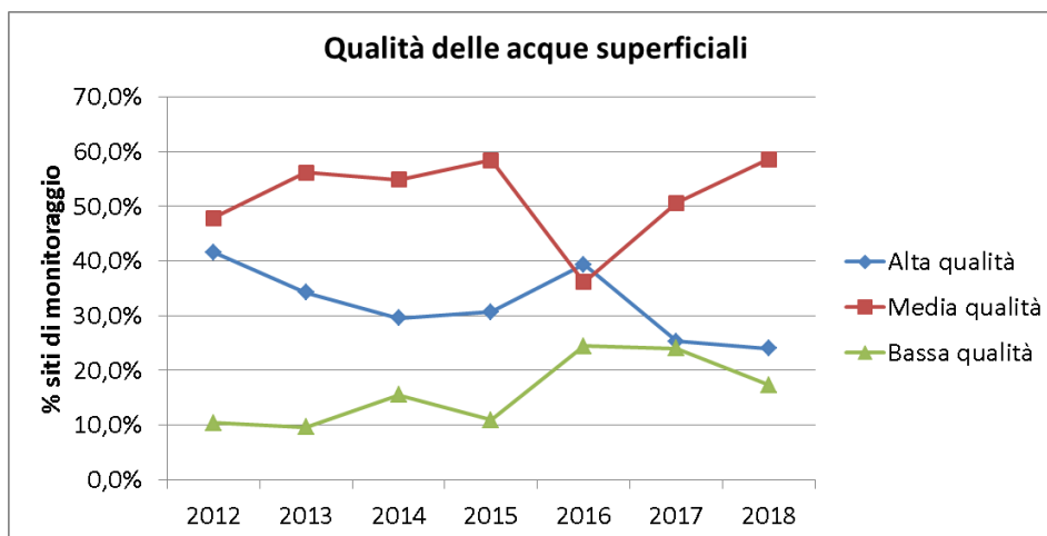
Figura 10. Evoluzione della qualità delle acque dolci superficiali per a presenza di Nitrati.
