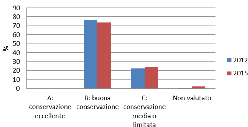
Figura 25. Valutazione dello stato di conservazione degli habitat non forestali in percentuale.
