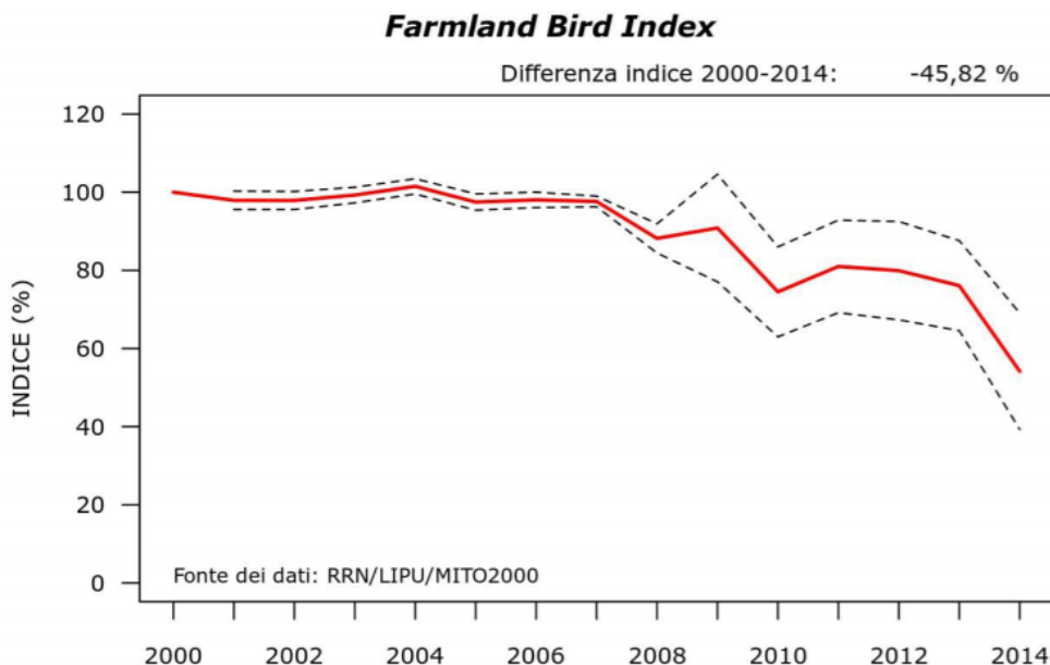
Figura 5. Evoluzione del Farmland Bird Index .
