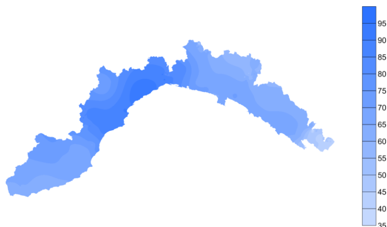
Figura 14. Stock di carbonio organico (ton/ha) nel periodo 2014-2016.
