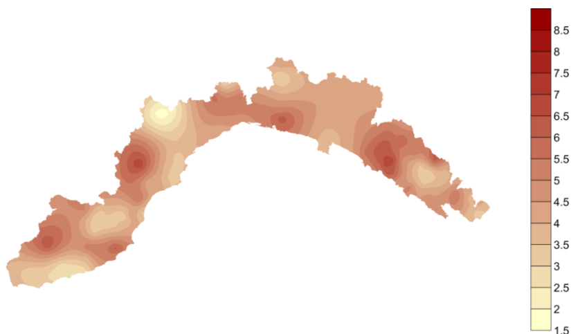
Figura 11. Mappa tematica della sostanza organica (%) riferita al periodo 2011-2013.
