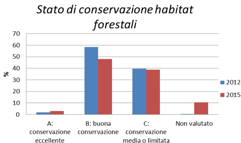
Figura 24. Valutazione dello stato di conservazione degli habitat forestali in percentuale.
