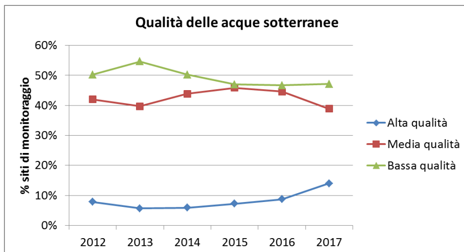
Figura 9. Evoluzione della qualità delle acque dolci sotterranee.
