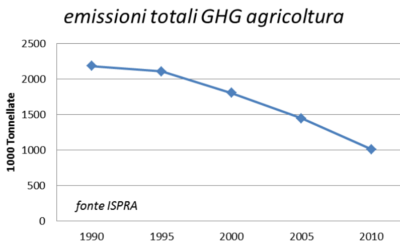
Figura 18. Emissione di gas a effetto serra in agricoltura in migliaia di tonnellate.
