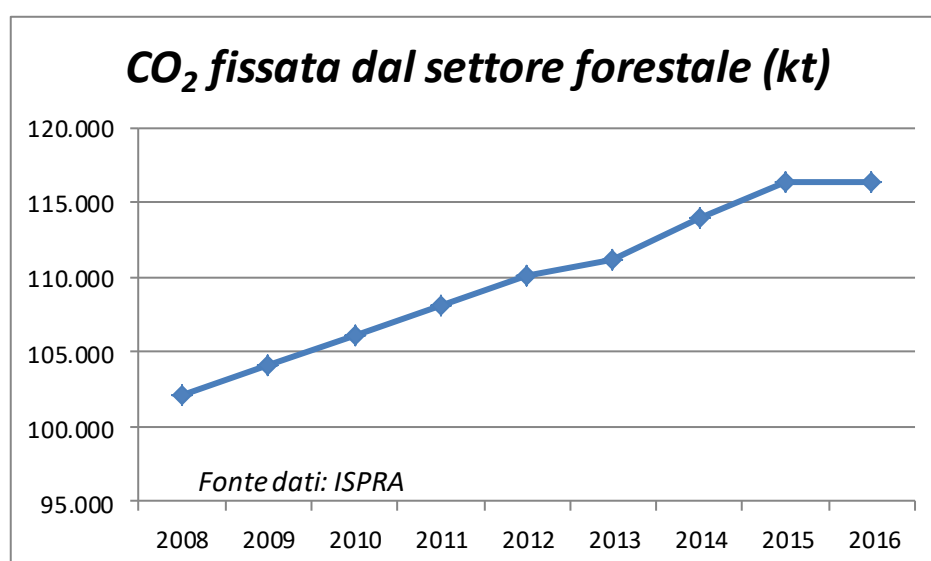
Figura 23. Evoluzione temporale della CO 2 fissata dal settore forestale (espressa in kt).
