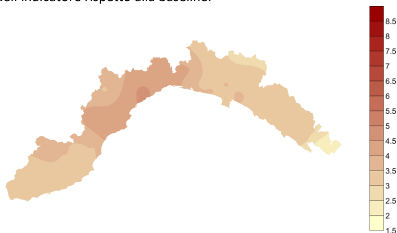
Figura 13. Mappa tematica della sostanza organica (%) riferita al periodo 2014-2016.
