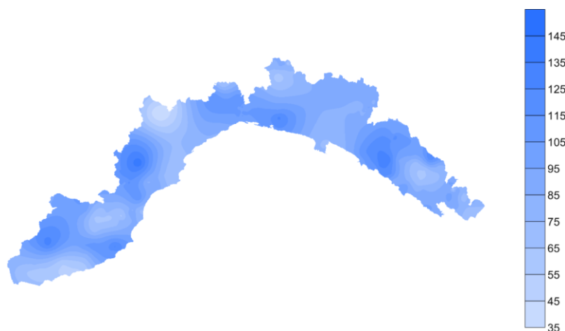
Figura 12. Stock di carbonio organico (ton/ha) nel periodo 2011-2013.
