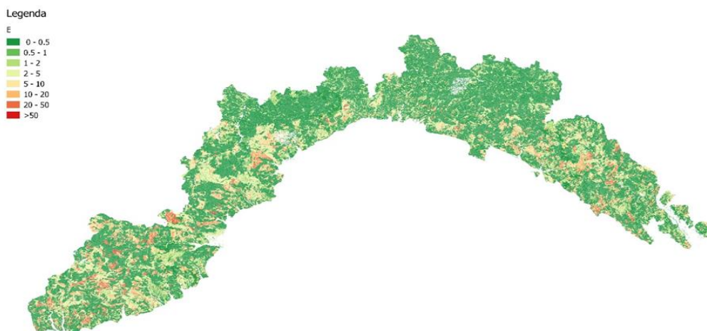
Figura 15. Tasso medio di perdita del suolo.
