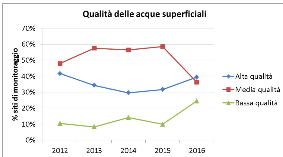
Figura 8. Evoluzione della qualità delle acque dolci superficiali.
